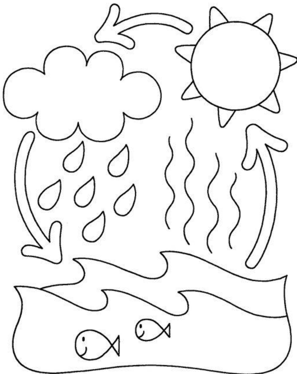
CICLO DELL'ACQUA
